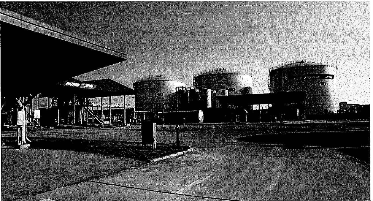
Kho Nhựa đường Puma do PEC làm tổng thầu EPC (Quy mô gồm 03 bồn (7000m 3 ) và các hạng mục phụ trợ như: Văn phòng, hệ thống công nghệ xuất nhập khẩu, điện tự động hóa, cấp thoát nước ...)
