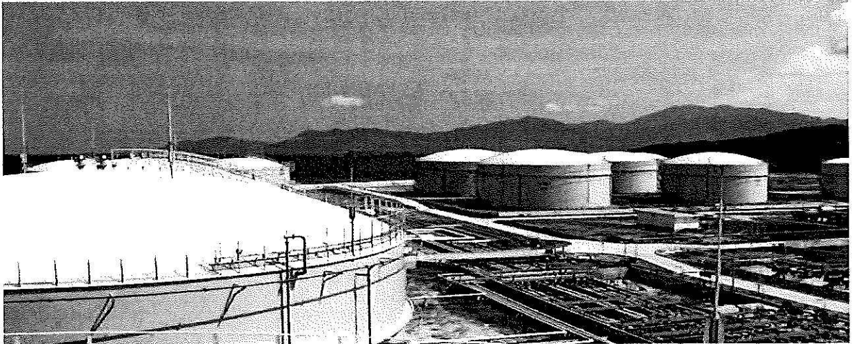
Bể chứa dầu cho Nhà máy lọc dầu Nghi Sơn do Công ty thiết kế khối bồn gồm 40 bồn thép
